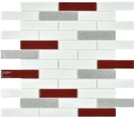
361CKM-9116 1500 tl +kdv 23 x 98 x 4 mm Plaka ebat : 30 x 30 cm Kutu : 1m 2 - 11 Plaka
