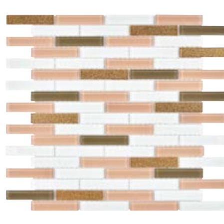
361CKM-9107 15 x 73 x 4 mm Plaka ebat : 30 x 30 cm Kutu: 1m 2 - 11 Plaka
